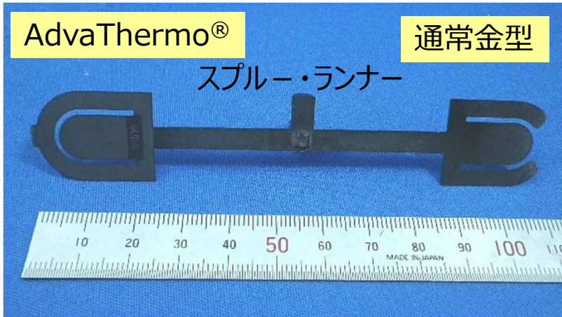
製品肉厚0.5mmt, 金型温度80℃
