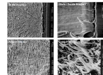
故障解析
