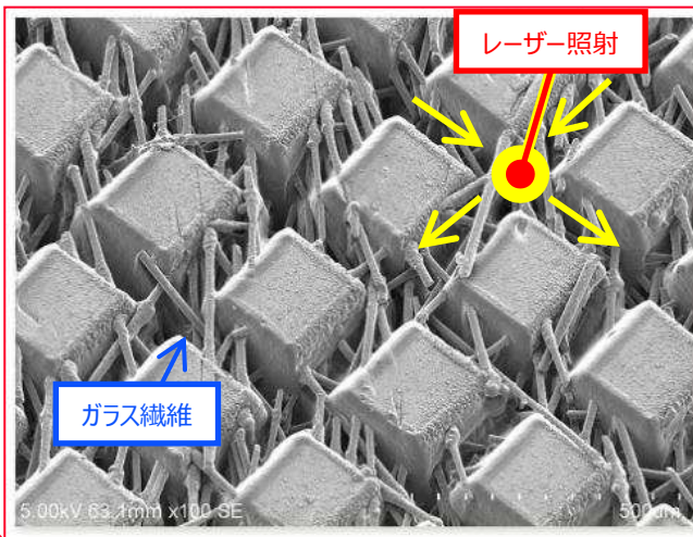
レーザー処理後の表面SEM写真
