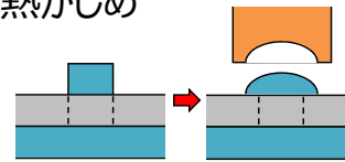
熱かしめ
