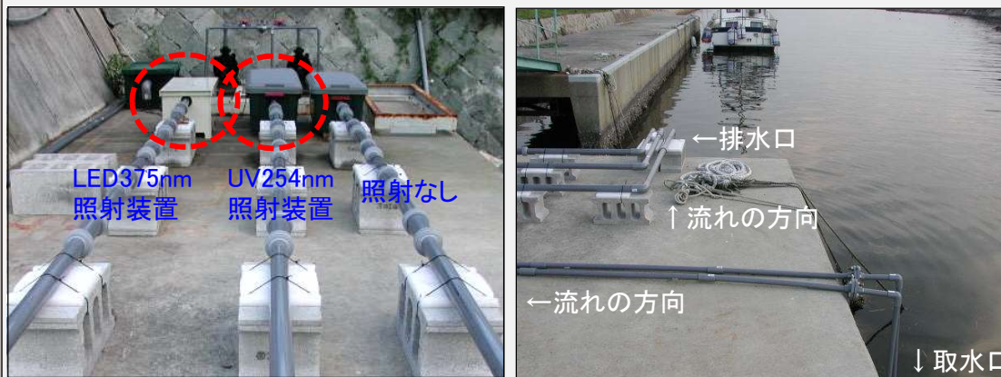
小型流水モデル水路の設置状況 (LED375nm、UV殺菌灯254nm、照射なし)
