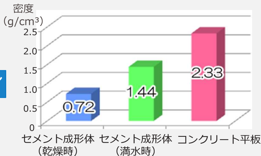
水に浮くセメント成形体
