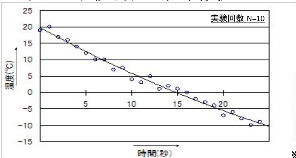
【 性能評価 (IH出力 1kW使用時) 】
