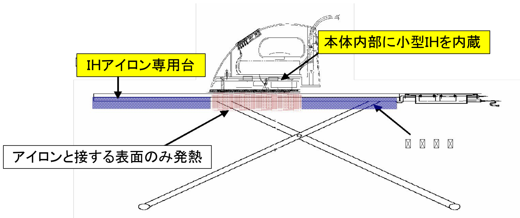
【 アイロンの構成図 】
