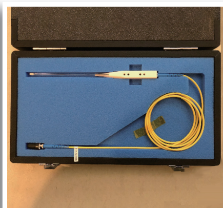
プリズム付き光電磁界プローブ
