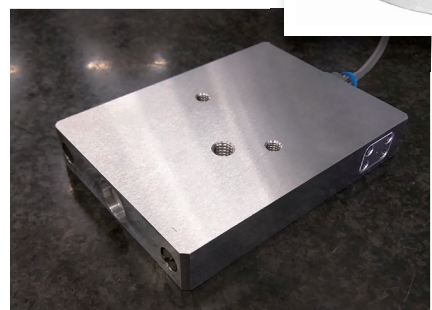
バキュームプリロード エアベアリング
