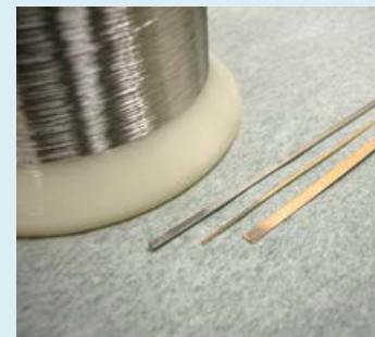
Precision rolling wire
